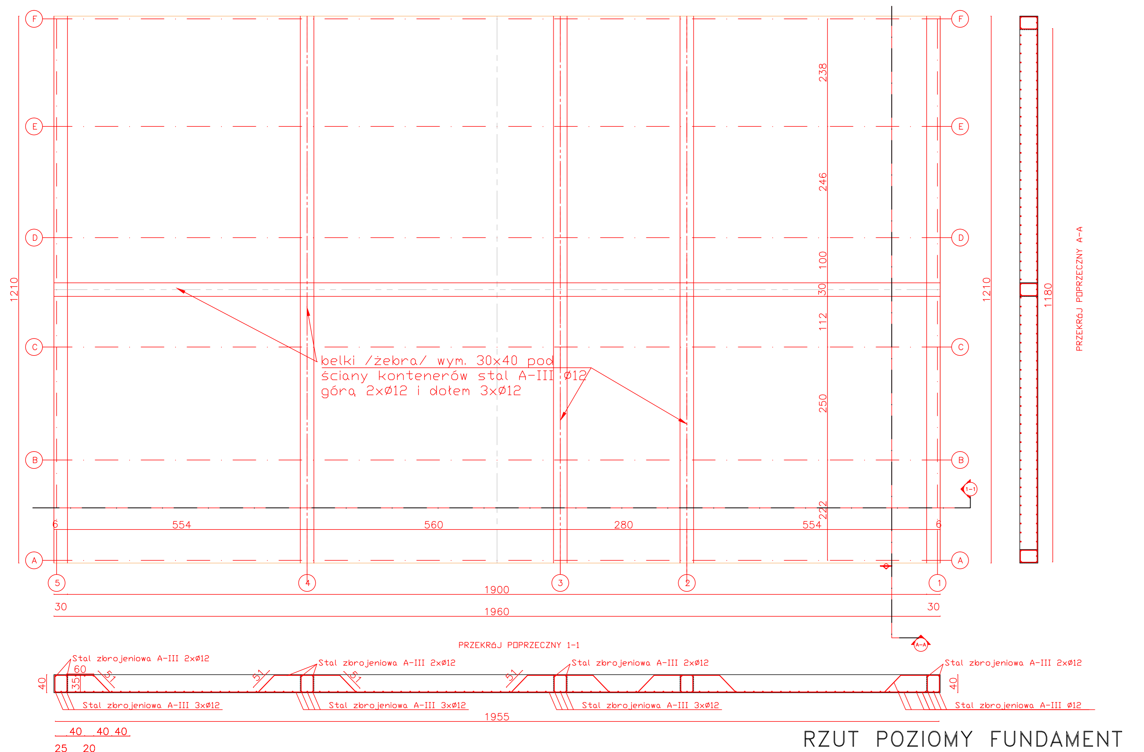
PŁYTA FUNDAMENTOWA ŻELBETOWA KRZYŻOWO ZBROJONA
